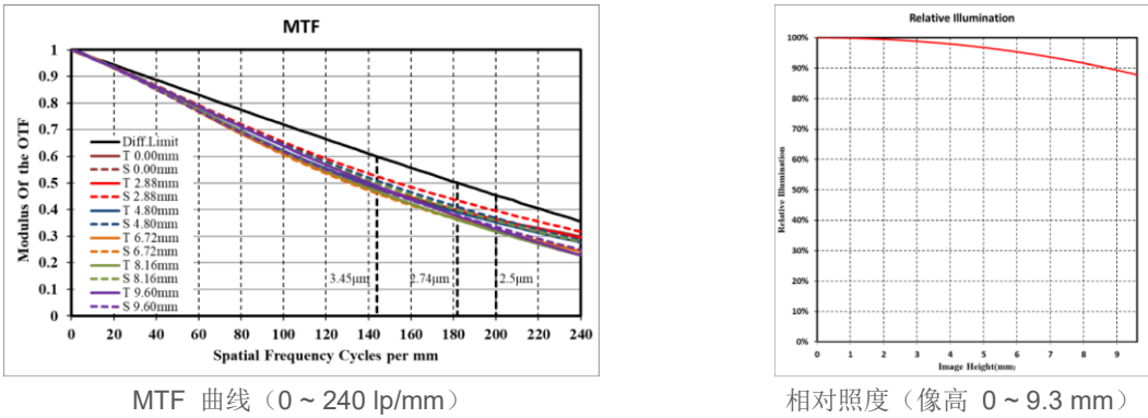
图 3-2 PRE-LF25 成像质量曲线
