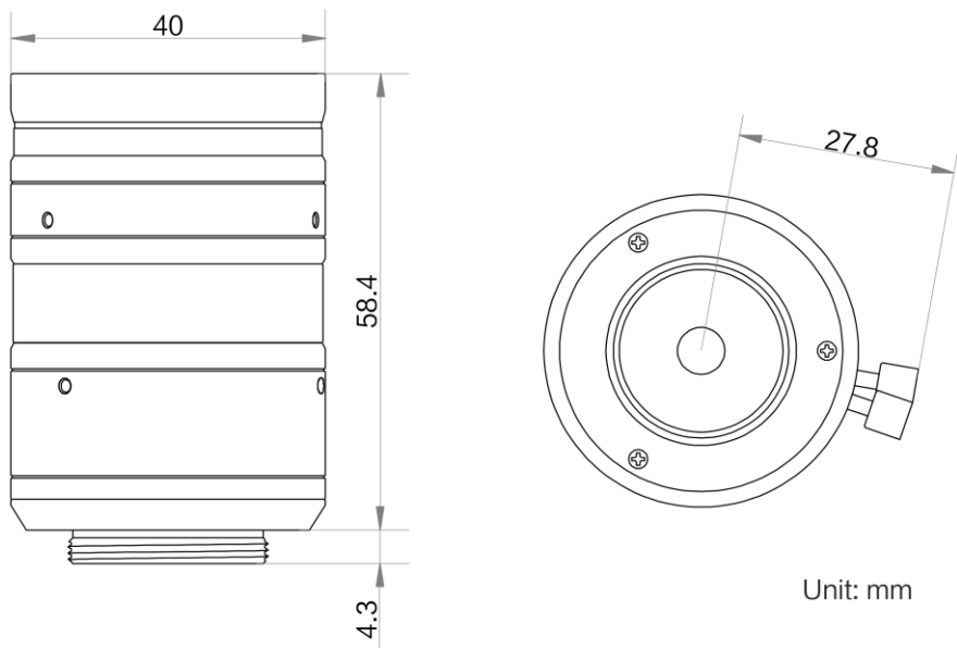
图 3-1 PRE-LF25 外形尺寸（单位：mm）
