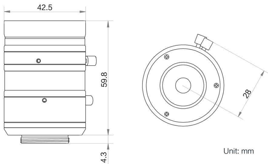
图 3-1 PRE-LF16 外形尺寸（单位：mm）
