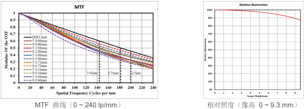
图 3-2 PRE-LF16 成像质量曲线
